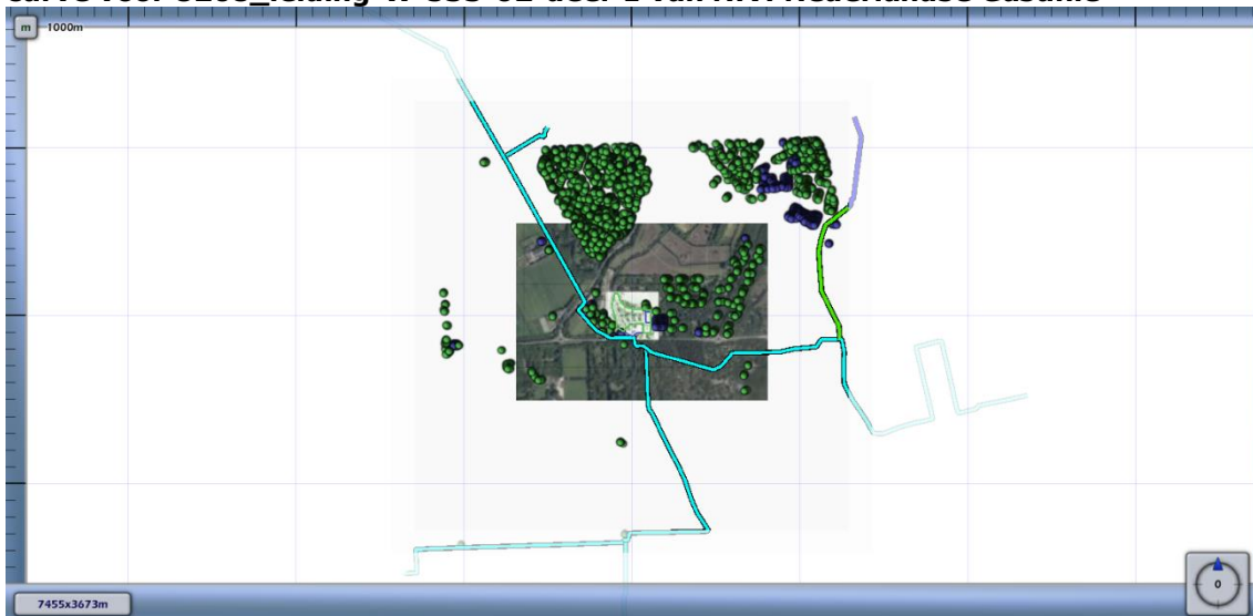
Figuur 4.2 Kilometer leiding behorende bij de maximale overschrijding van de FN-curve voor 8208_leiding-W-533-02-deel-1 van N.V. Nederlandse Gasunie
