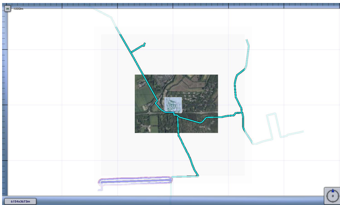
3.4 Figuur 3.4 Plaatsgebonden risico voor 8208_leiding-W-533-12-deel-1 van N.V. Nederlandse Gasunie
