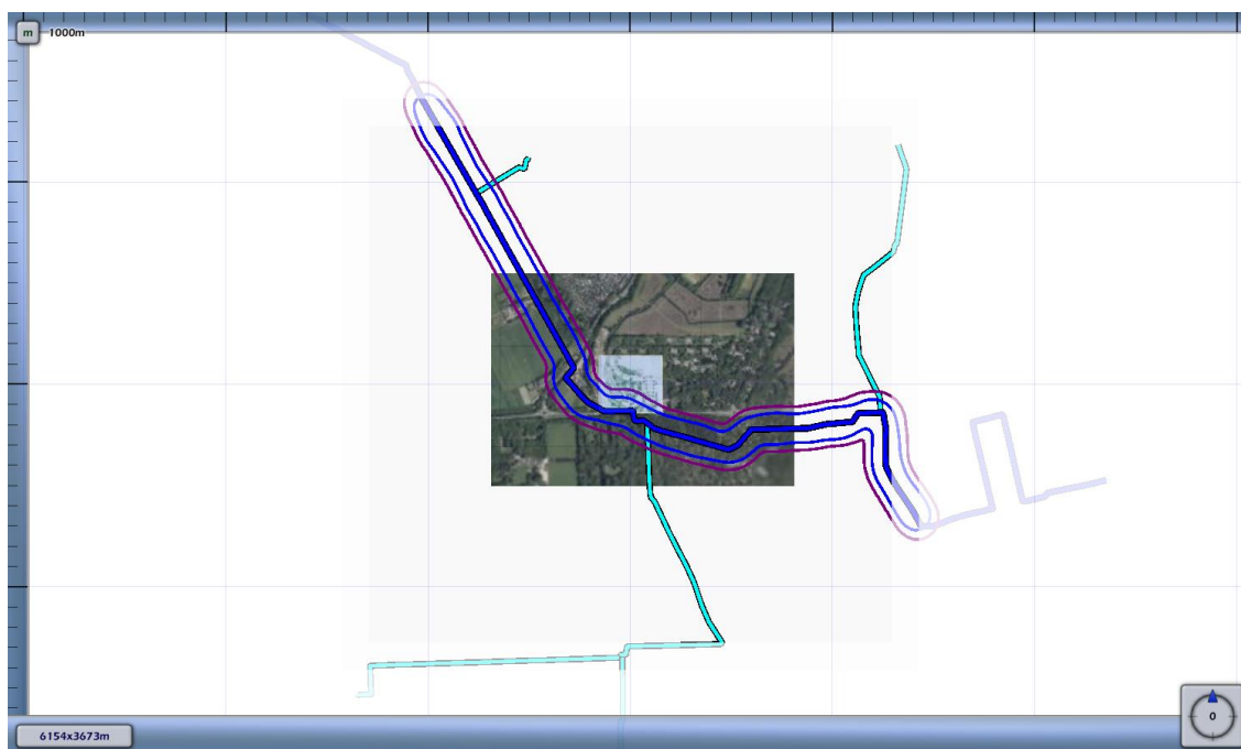
3.2 Figuur 3.2 Plaatsgebonden risico voor 8208_leiding-W-533-02-deel-1 van N.V. Nederlandse Gasunie
