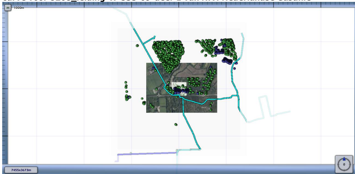
Figuur 4.3 Kilometer leiding behorende bij de maximale overschrijding van de FN-curve voor 8208_leiding-W-533-09-deel-1 van N.V. Nederlandse Gasunie
