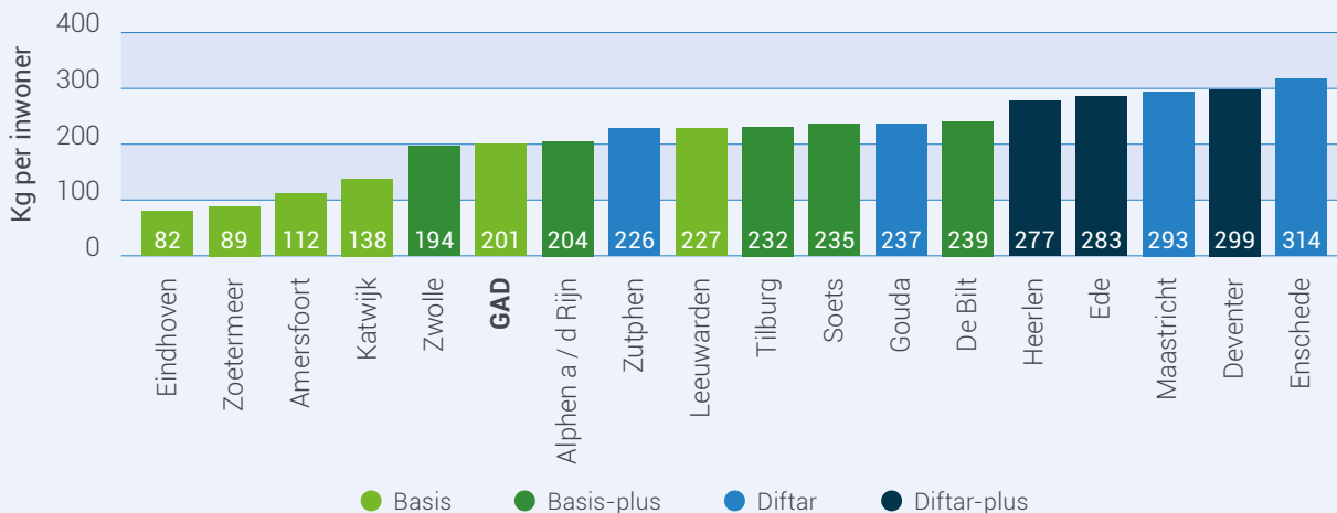
Figuur 8 - CO2-reductie
