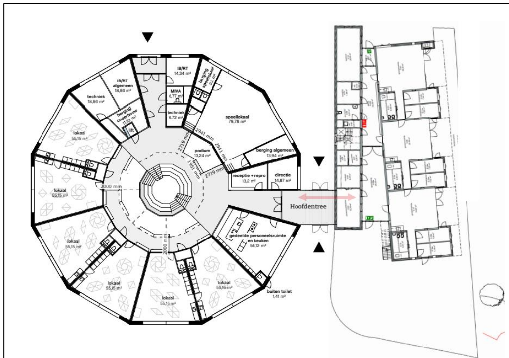
Vloerontwerp (alleen het ronde deel tot en met de hoofdentree zal nieuwbouwd worden)
